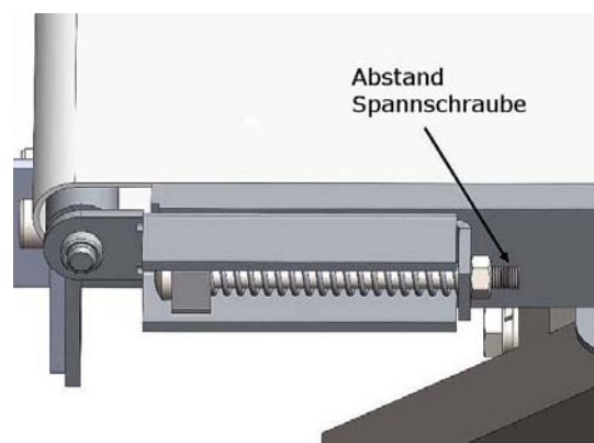
Abb. 36: Position der Spannschrauben
