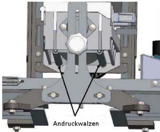
Abb. 25: Andruckwalzen
