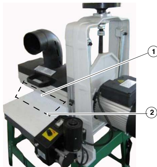
Abb. 2: Gefahrenbereiche
