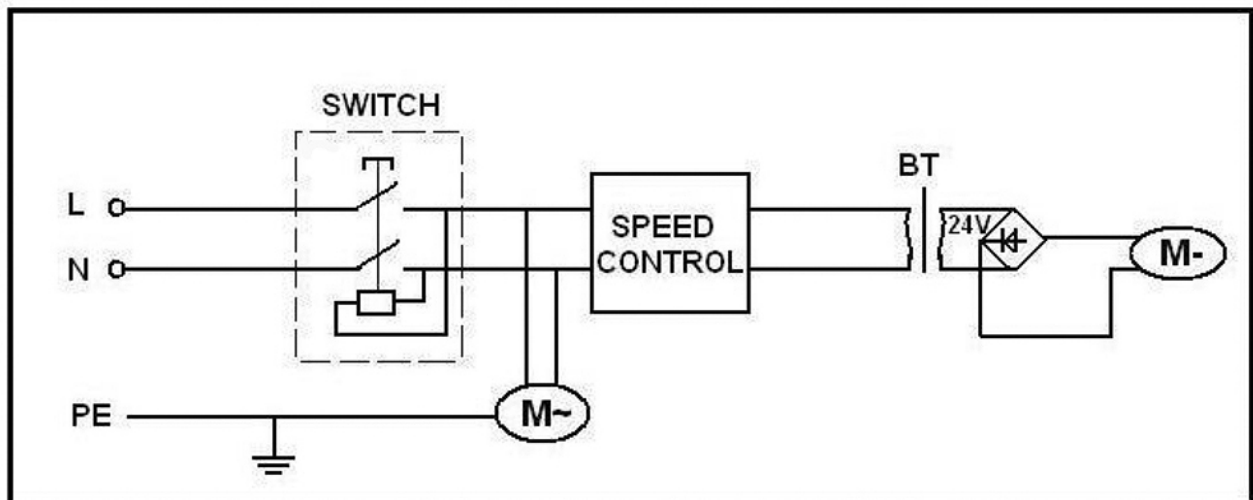
Abb. 39: Elektro-Schaltplan ZSM 405
