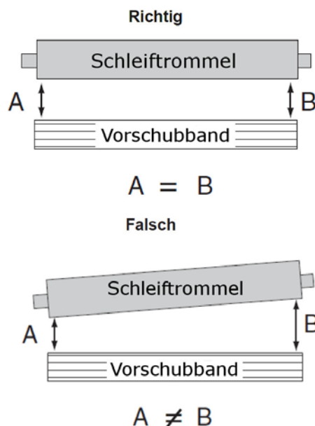
Abb. 30: Parallelität von Vorschubband und Schleiftrammel
