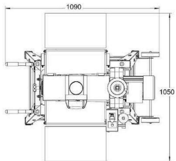
Abb. 6: Platzbedarf der Maschine
