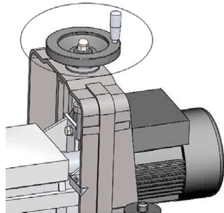
Abb. 15: Handrad montieren
