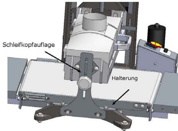
Abb. 33: Vorschubband austauschen
