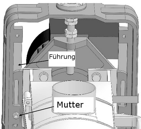
Abb. 28: Führungsseiten lösen
