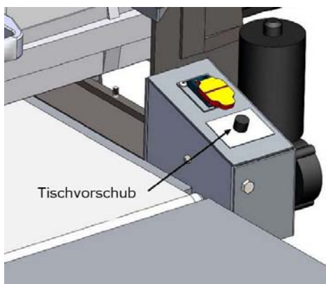
Abb. 18: Vorschubgeschwindigkeit einstellen
