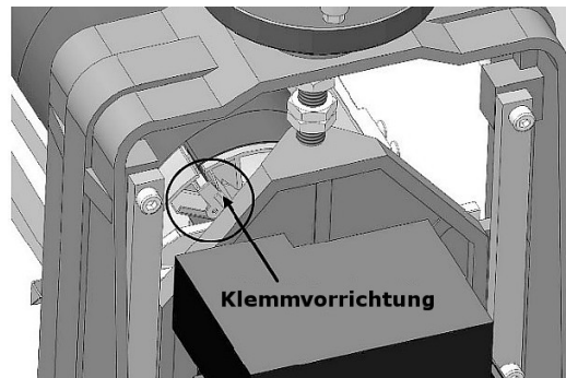
Abb. 21: Klemmvorrichtung rechts
