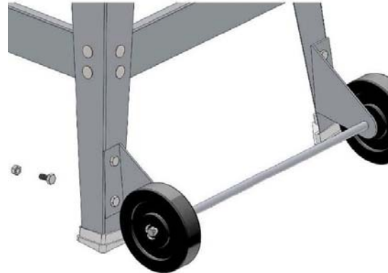
Abb. 11: Transporträder der Maschine montieren
