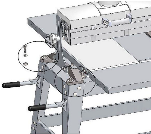
Abb. 13: Maschine auf Untergestell montieren
