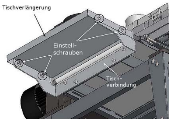
Abb. 14: Tischverlängerung montieren
