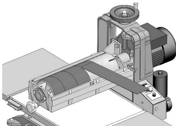
Abb. 23: Schleifpapier aufwickeln
