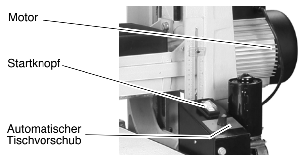
Abb. 17: Starten der Maschine
