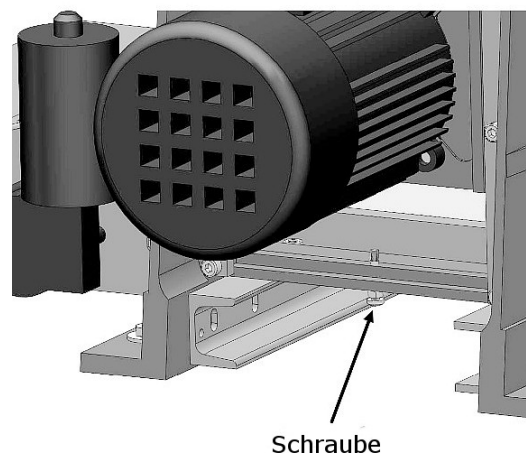
Abb. 27: Einstellschraube Höhenanschlag
