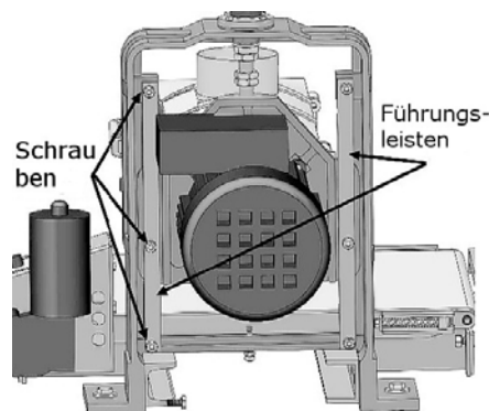
Abb. 29: Führungsseiten einstellen
