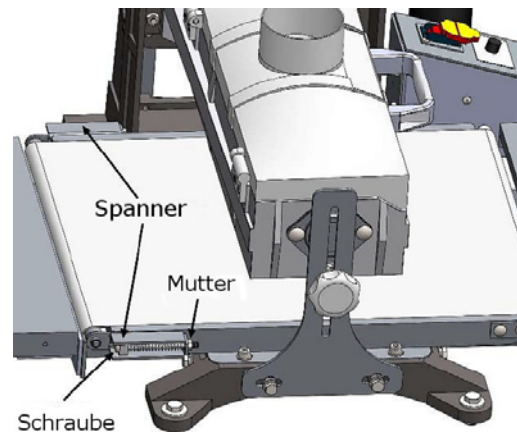
Abb. 35: Vorschubband spannen
