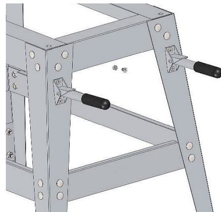
Abb. 12: Transportgriff der Maschine montieren
